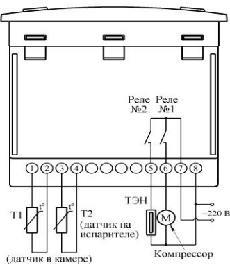
Рис. 1. Схема подключения устройства
